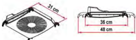
Turbo Kit auf Hymer-Dachhaube, 50x70 cm
