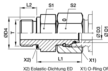
X2) Elastische-Dichtung ED X1) O-Ring OR
