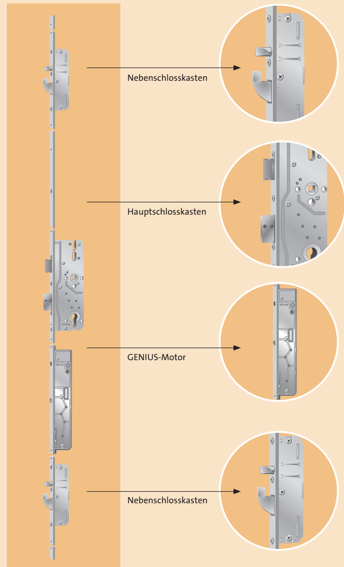
Abbildung zeigt AS 2600 EA
