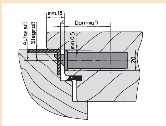
Überfälzte Holztür, 4 mm Falzlufte, Türverschluss mit 20 mm Stulpbreite.
