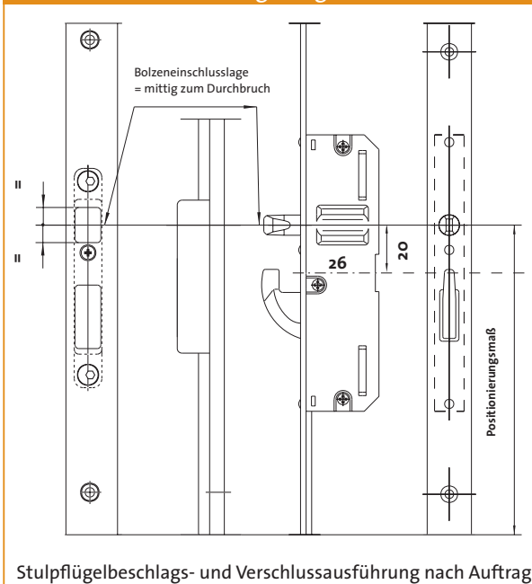
Abb. 1 Einbau des Stulpflügelbeschlages zur Mehrfachverriegelung
