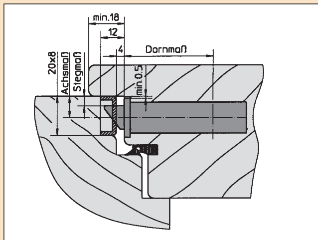
Überfälzte Holztür mit Euro-Falz 20 x 8 mm.
