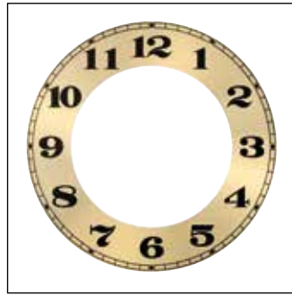
Zahlenreif Nur solange der Vorrat reicht! Goldfarben. Mit arabischen Ziffern und Minuteneinteilung am äußersten Kranz. Aus Aluminium mit der Stärke 0,4 mm. Außen-Ø 127 mm, Innen-Ø 80 mm. 341403 11,50 Außen-Ø 150 mm, Innen-Ø 98 mm. 341404 11,50
