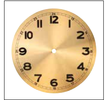
Zifferblatt Nur solange der Vorrat reicht! Ø 267 mm, arabisch, Messing, gelb, Stärke 0,5 mm, Mittelloch 12,0 mm. 341410 22,30
