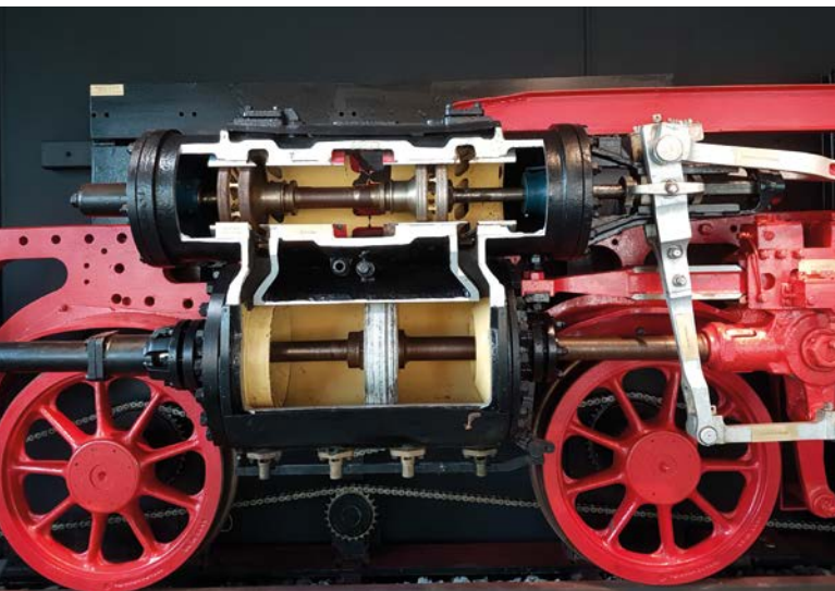
Der aufgeschnittene Zylinderblock der 01 1080 zeigt die Bewegung von Kolben und Schieber.
