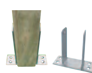
Pfostenträger (ähnli. Abb.) verzinkt, zum Aufschrauben (ohne Schrauben)
