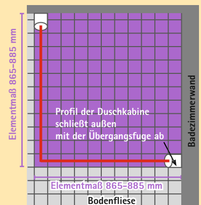
Beispiel: Garant Drehtür mit Seitenwand
