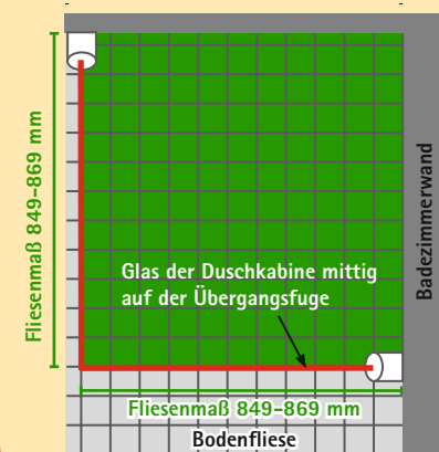
Beispiel: Garant Drehtür mit Seitenwand
