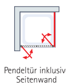
Sunny Pendeltür inklusive Seitenwand, 2-teilig • 5 mm starkes Sicherheitsglas (ESG) • Höhe: 1800 mm; verkürzte Seitenwand: 1550 mm mit Stabilisationsbügel: 1850 mm • Öffnet nach innen und außen
